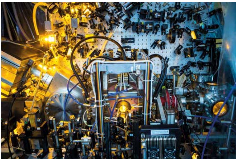
Detail van de Bose-Einstein opstelling van hoogleraar Peter van der Straten bij het Debye Instituut voor nanomaterialen, UU.
